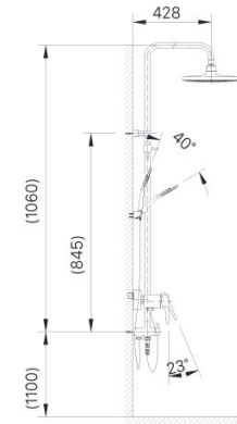
BFV-50S-5C Giá: 12.290.000 VNĐ Áp lực nước cấp 0.07-0.75MPa
