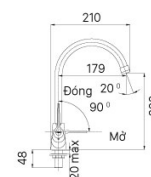
SFV-17 Giá: 760.000 VNĐ
