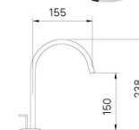
LFV-7100B Giá: 8.120.000 VNĐ
