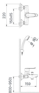
BFV-2013S Giá: 2.600.000 VNĐ
