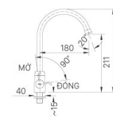
SFV-21 Giá: 1.200.000 VNĐ
