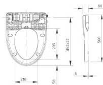
BẢNG KẾT HỢP NẮP CW-S15VN
